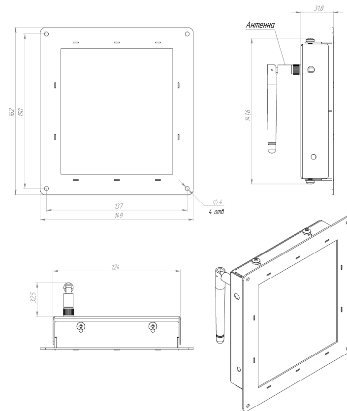
Рисунок 1 Блок управления светильниками LCS-01
